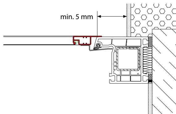
schemat 2
