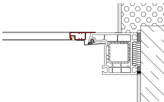
schemat 1
