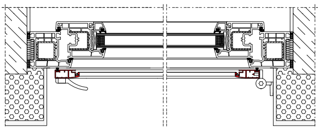
montaż na ścianie we wnęce
