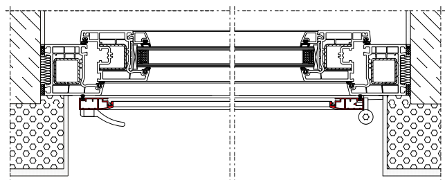
montaż na ramie okna we wnęce
