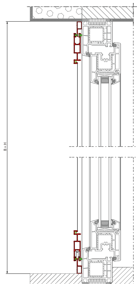
Moskitiera ramkowa przesuwna z ramą montaż we wnęcie
