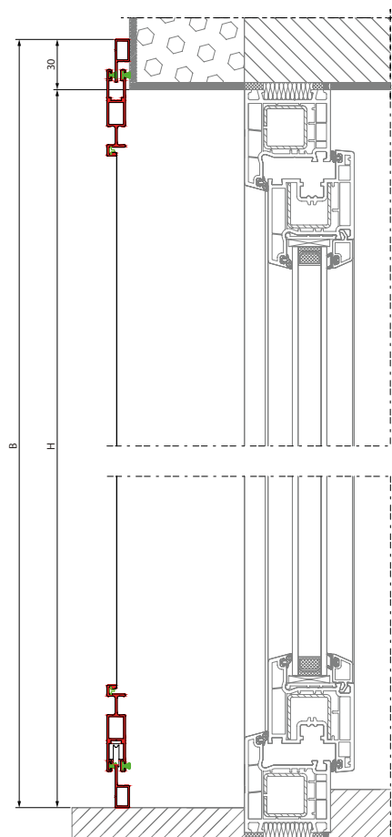
Moskitiera ramkowa przesuwna bez ramy montaż na mur
